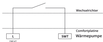
Abbildung 9 (links): Wärmepumpe an Kontakt von Wechselrichter (Quelle: ait)
