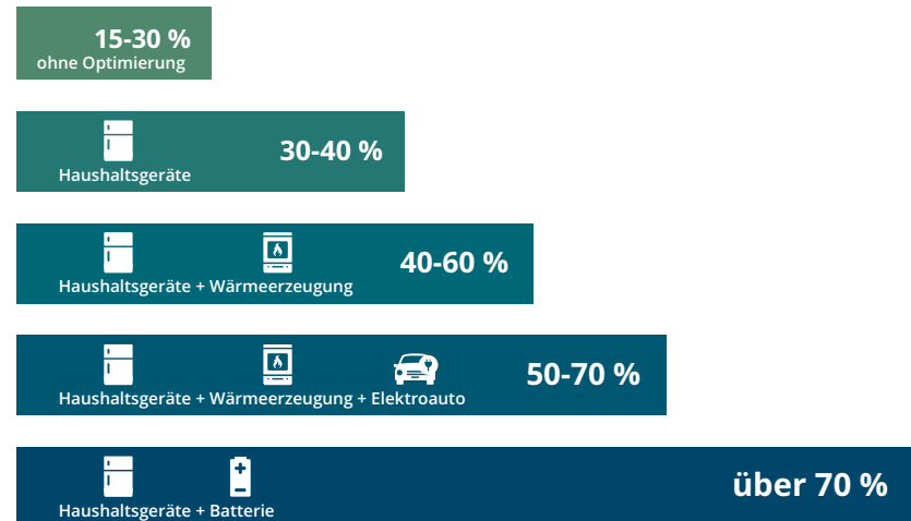
Abbildung 8: Richtwerte für erreichbaren Eigenverbrauchsanteil in Abhängigkeit der optimierten Gerätegruppen
