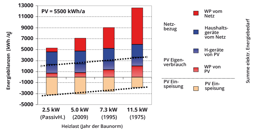
Abbildung 4: Eigenverbrauchsanteile im Wärmepumpenbetrieb bei einer PV-Anlage mit 5'500 kWh/a Ertrag. 40 bis 60 % Eigenverbrauch sind möglich, aber es bleibt ein grosser Strombezug im Winter. Quelle: www.zsw-bw.de/uploads/media/OTTI_Dezentrale-PV_Binder-Kelm_2012.pdf
