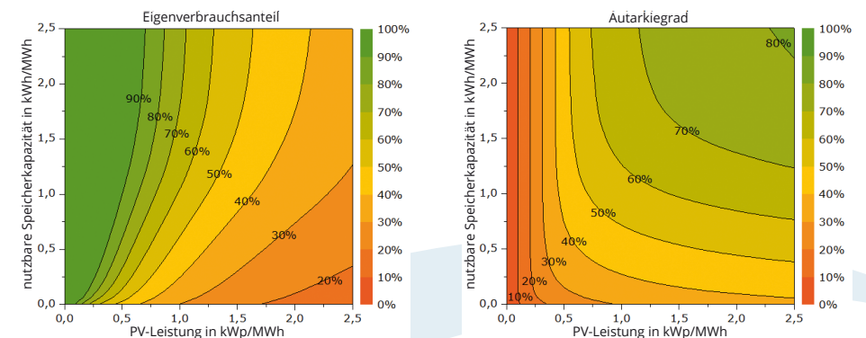
Abbildung 7: Eigenverbrauch in Abhängigkeit von Batterie- und PV-Anlagegrösse, siehe auch www.volker-quaschnig.de/artikel/2013-06-Dimensionierung-PV-Speicher/index.php
