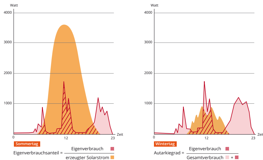
Abbildung 1: Eigenverbrauchsanteil versus Autarkie: Sommertag: Eigenverbrauch 15 %, Autarkie 70 %; Wintertag: Eigenverbrauch 60 %, Autarkie 20 %
