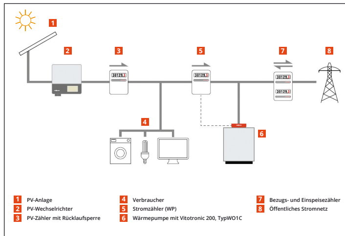
Abbildung 11: Wärmepumpen-Steuerung unter Einbezug Solarstrom von Viessmann
